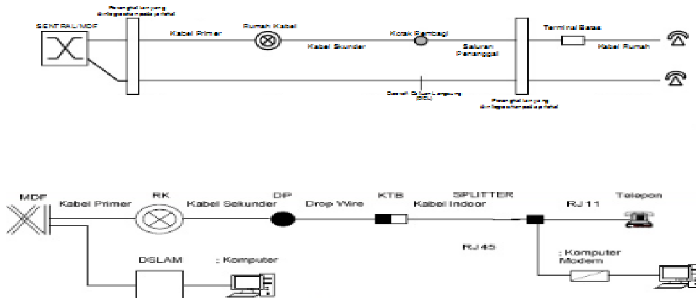
Gambar 1.7. Konfigurasi Jarlokat Tidak Murni
