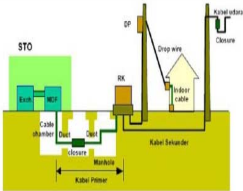
Gambar 1.1 Model Infrastruktur Jarlokat Primer-Sekunder
